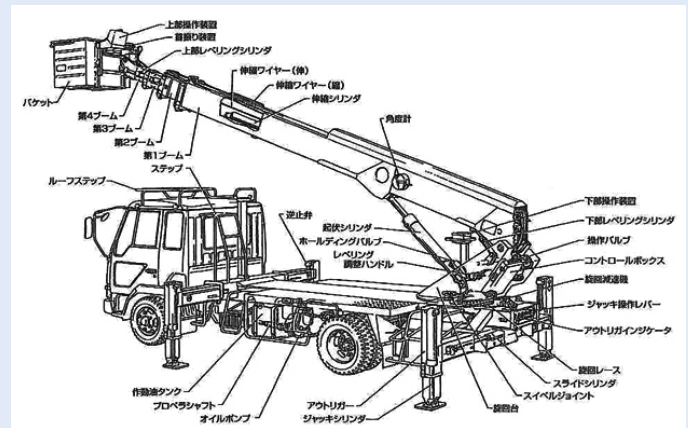
伸縮ブーム型高所作業車
